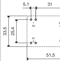
Вид со стороны выводов
