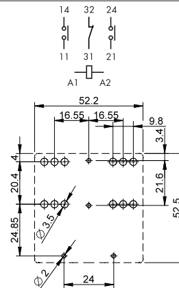
Вид со стороны выводов
