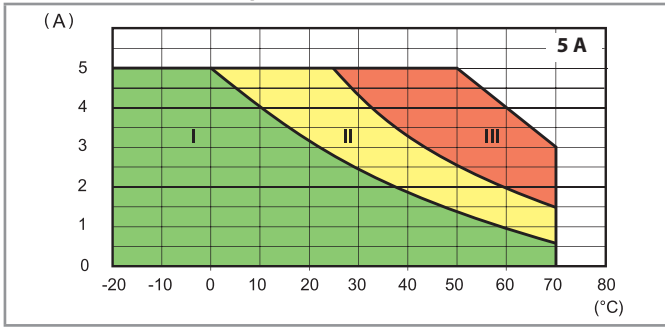
L77-1 Зависимость тока выход. цепи от температуры 77.01.x.024.805x при 32 В DC
