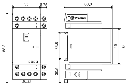
Тип 22.34 + 022.33/022.35 Винтовой клеммы
