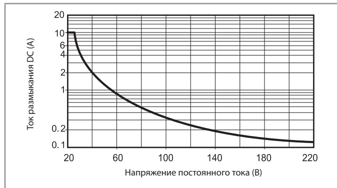
Н 8A - Макс. отключающая способность DC1
