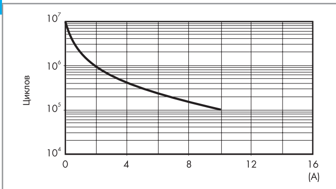
Н 8A - Электрическая долговечность (AC) при ном. нагрузке
