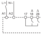
Схема подключения (без сигнала START)
