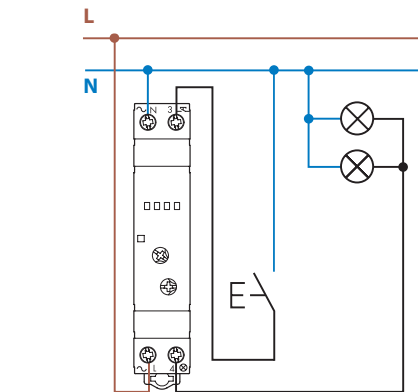
Тип 15.81 - 3-проводное соединение
