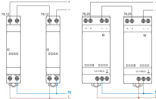
последовательное соединение
