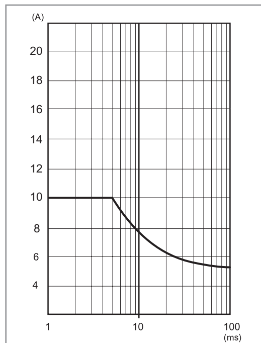
P78-9 Зависимость пикового тока на выходе от времени (78.1D)
