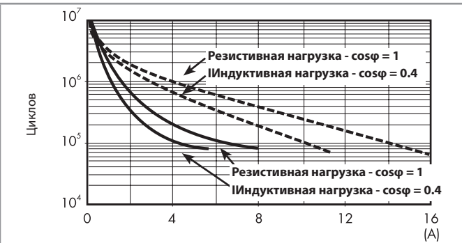
F 38 - Электрическая долговечность (АС) при ном. нагрузке, 1 полюс 16 А и 2 полюса 8 А
