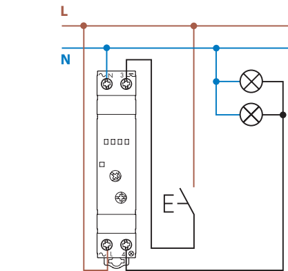
Тип 15.81 - 4-проводное соединение
