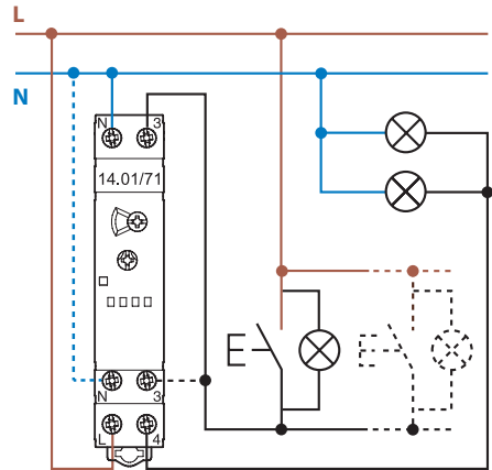
4-проводное соединение
